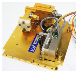
874 GHz レーザー
